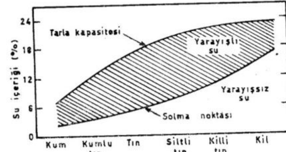
řekil 4.18: Farklı tekstüre sahip topraklar için tipik su tutma kapasiteleri ve yarayıřlı su düzeyleri (Foth ve Turk, 1972).
